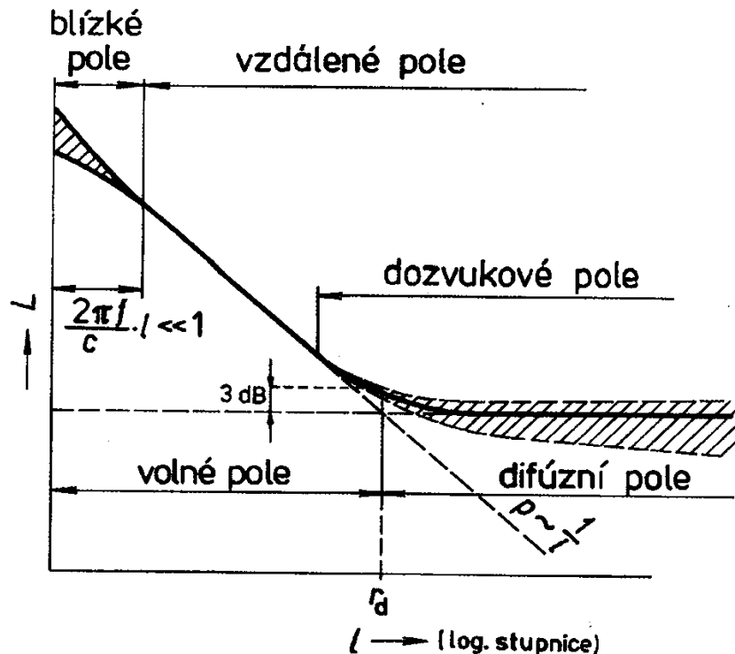
Obr. č. 1: Druhy akustických polí [L20]
