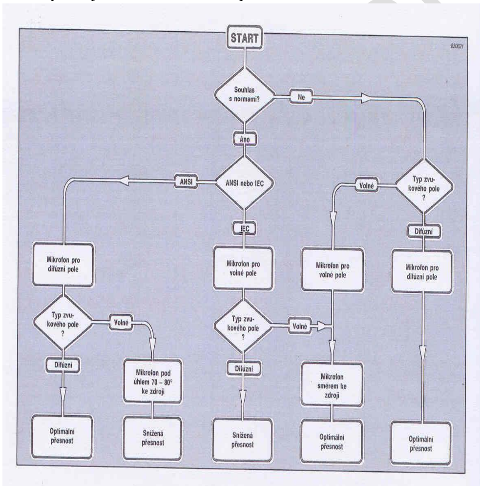
Obr. č. 2: Postup pro správné měření jednotlivých polí [L21]
