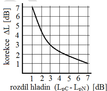
Obr. č. 3: Korekce na hluk pozadí
